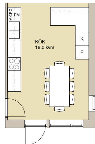
PLANLÖSNING VID TILLVAL AV BARKÖK
